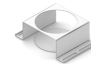
RA-Z009 GASFLASCHEHALTER (3/7)
